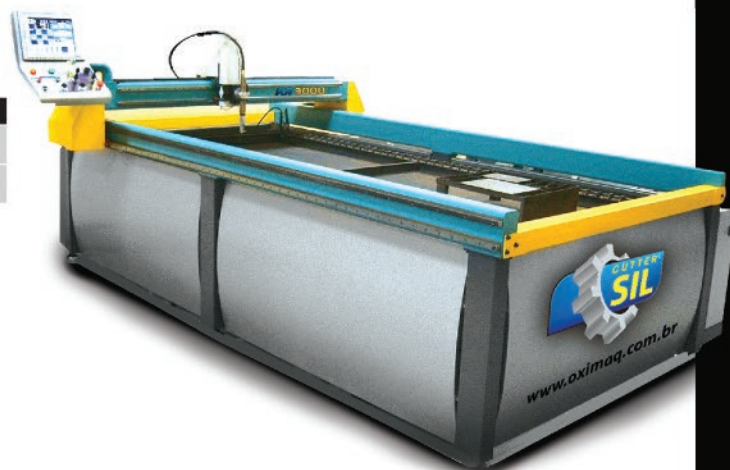
MÁQUINA CORTE ÓPTICA AUTOMATIZADA PARA PLASMA OU OXICORTE COM 2 CABEÇOTES - SEM MAÇARICO SEM TOCHA 02.053.0216
